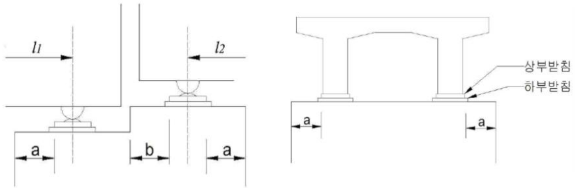
【그림 3.2.18】 받침의 끝에서 거더 끝단까지의 거리(a 및 b)의 값
